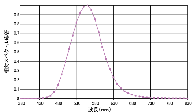
Fig.4 HD2021T6、HD2021T7、HD2021T7.2の相対スペクトル応答
