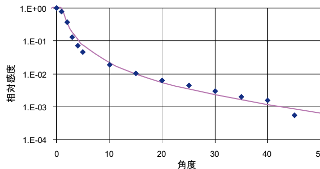
Fig.5 HD2021T7の相対角応答
